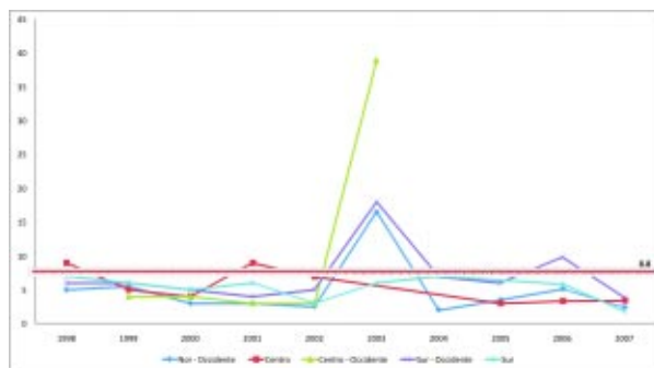
Gráfica 2.40. CO Concentración en ppm (Máximos Anuales de Datos Diarios), 1998-2007. Fuente: Secretaría Distrital de Ambiente, Informe Anual Consolidado sobre niveles de concentración de Contaminantes 2005,2006. Informe Mensual de Calidad del Aire de Bogotá Diciembre de 2007. Cálculo: UN - HABITAT/ COLOMBIA. Resolución 601 Norma (Anual): 8.8 ppm
